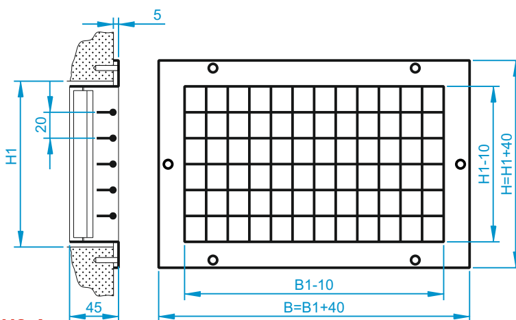
РА2-А, РН2-А
