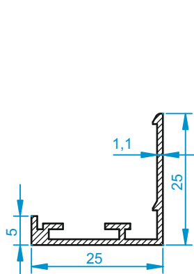
Сечение профиля рамки РА2, РА3
