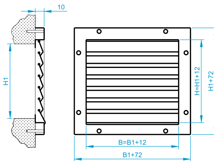
КОН2
