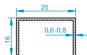
Сечение профиля перемычки
