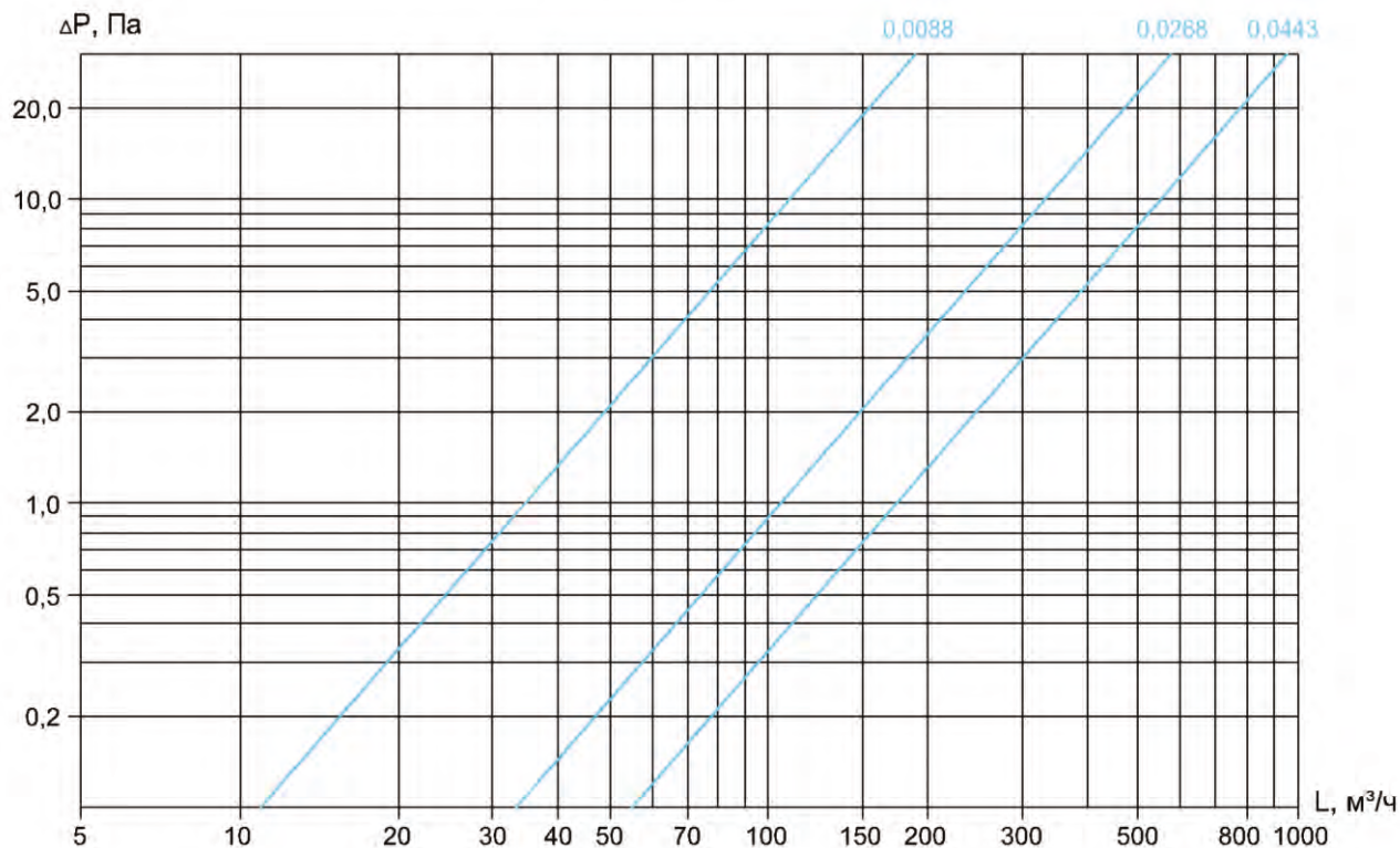
Потери давления для решеток PC5турбо-П, PC5ПНтурбо-П
