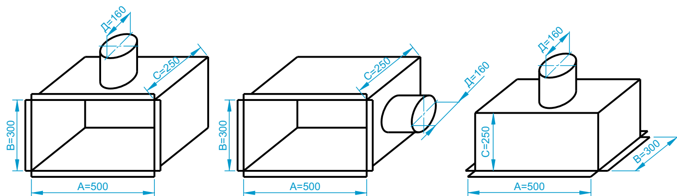
УП2-Б-500х300х250-160
