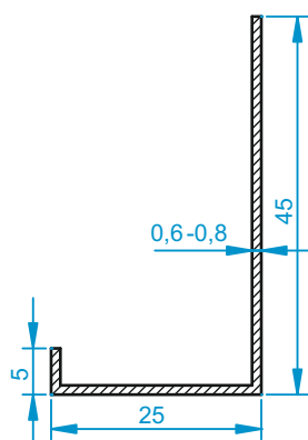
Сечение профиля рамки РН2-А
