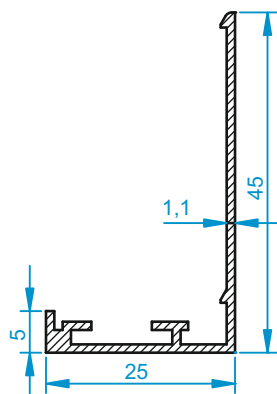
Сечение профиля рамки РА2-А
