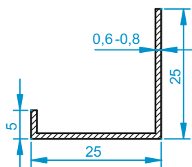
Сечение профиля рамки РН2, РН3
