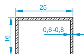
Сечение профиля перемычки РА2, РА3, РА2-А
